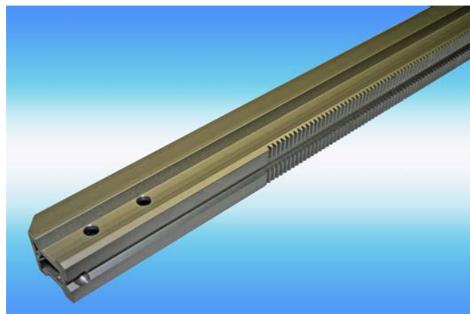
Rechthoekige tandheugel t.b.v. kolomboormachine voor de beton industrie
