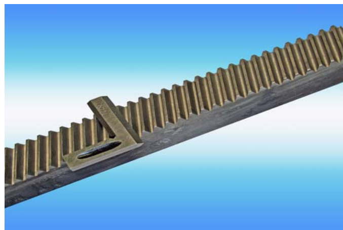
Schuin vertande tandheugel t.b.v. papier industrie
