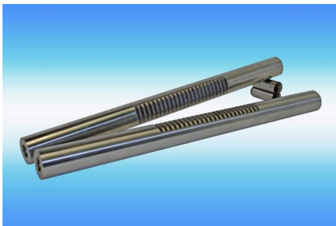
Ronde tandheugel t.b.v. stuurstang automotive industrie
